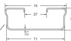
Perfil Del Riel Macho
