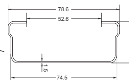
Perfil Del Riel Hembra
